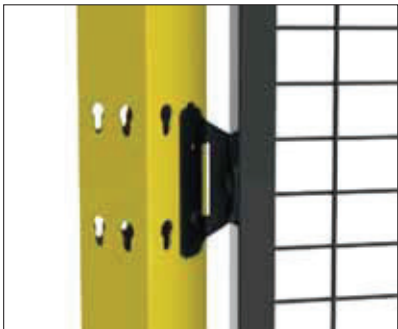
T01-01 調節角度金屬配件 (0-180°) 安裝角度最大為180°，需要以90°以外的角度安裝時，使用此配件
